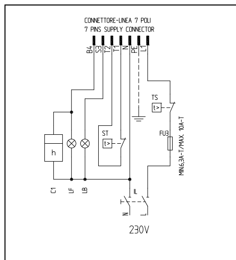
Рис. 28 - 7-х полюсные соединительные разъемы
