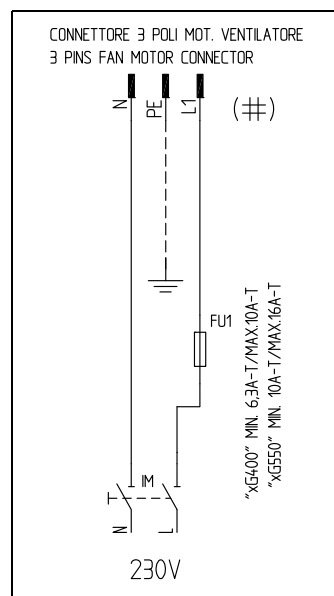
Рис. 31: 3-х полюсный соединительный разъем электродвигателя для NG/LG/NGX400
