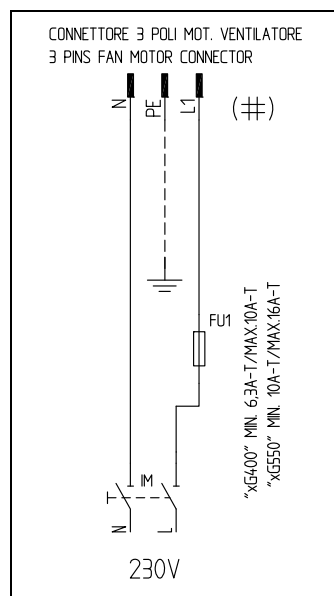
Рис. 29 3-х полюсные соединительные разъемы электродвигателей для NG/LG/NGX400
