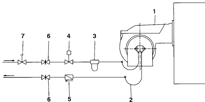
Fig. 4 - Sistema bitubo
