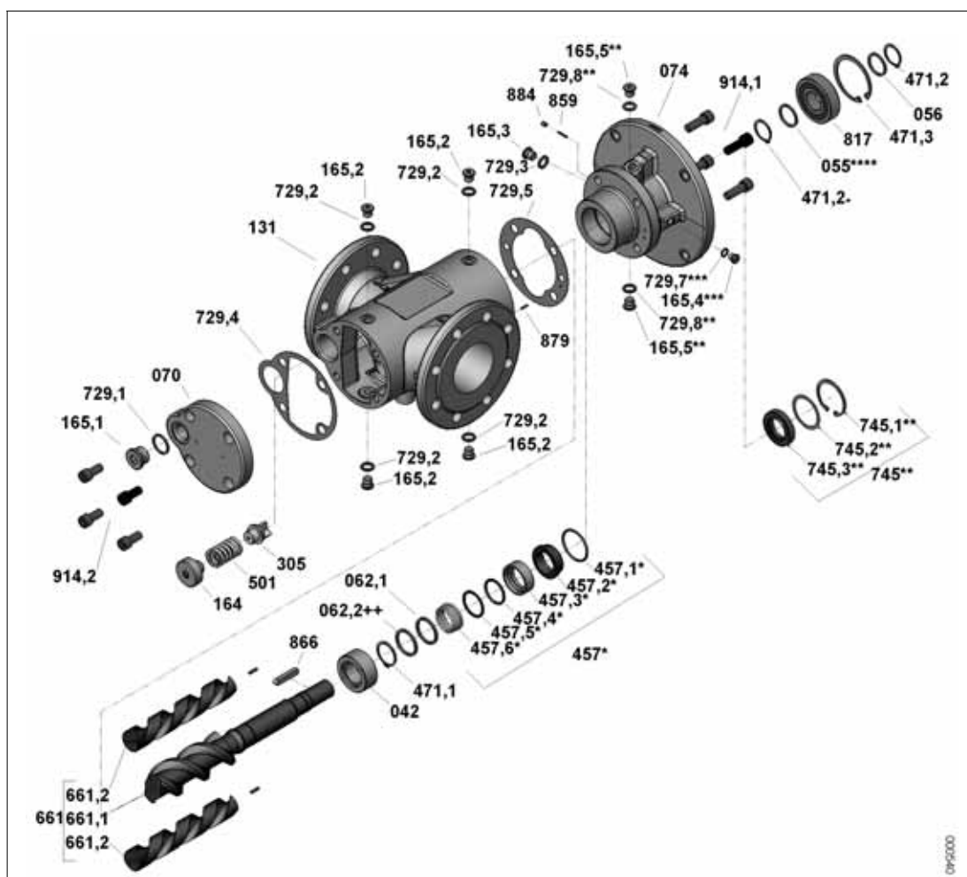
Рис. 2 Разнесенное изображение К 5 – 660
