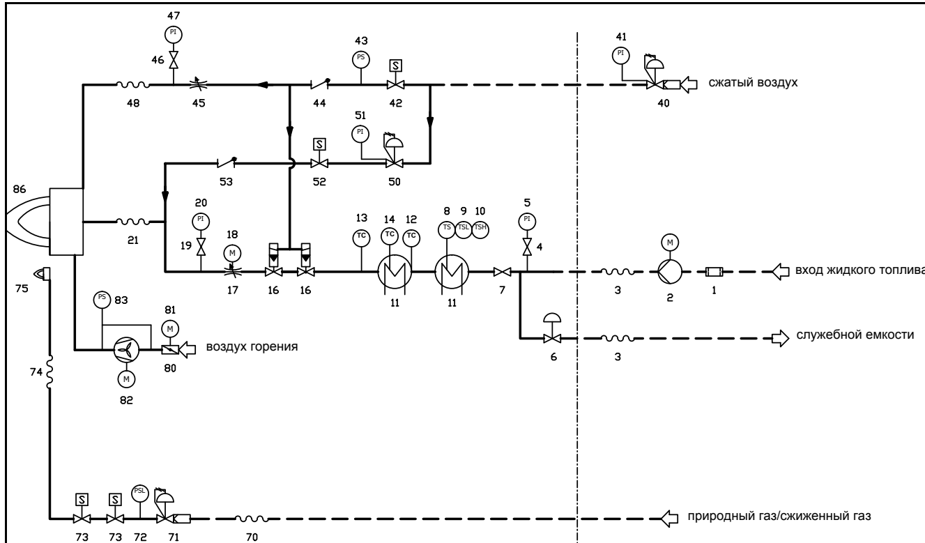
Рис. 5 - 3I2D-03 v5 – Гидравлическая схема
