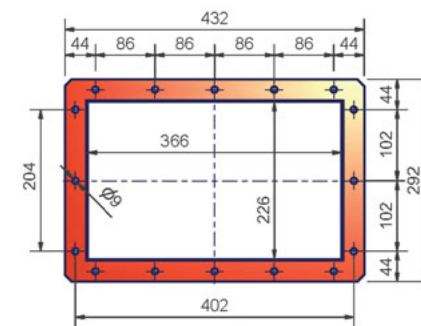
Controflangia e flangia canale aria
