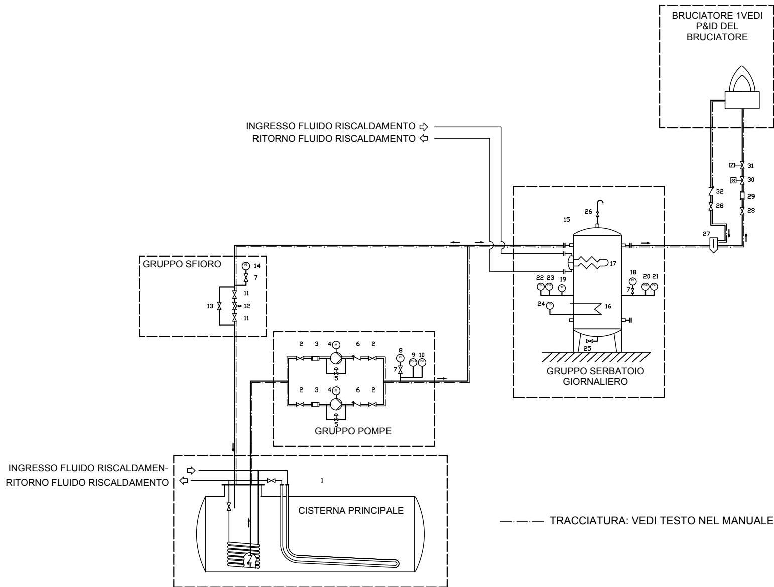
Fig. 6 - 3ID0023 v2 - Schema idraulico - Configurazione per un solo bruciatore
