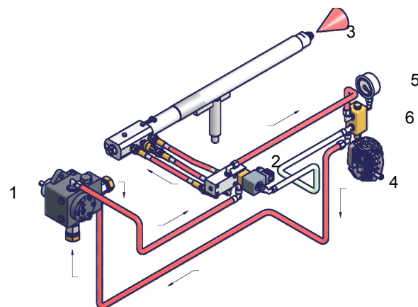
Fig. 20 - Alta fiamma
