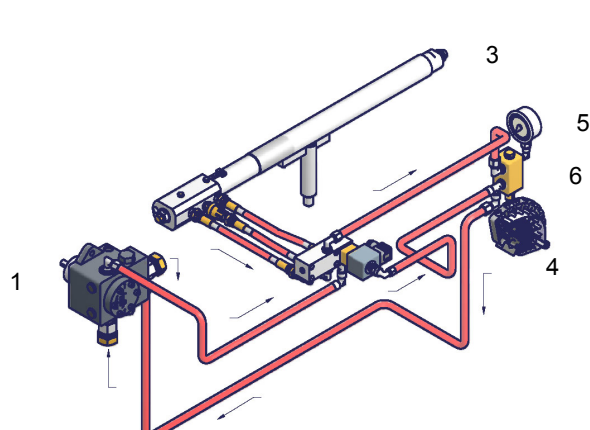
Fig. 18 - Preventilazione
