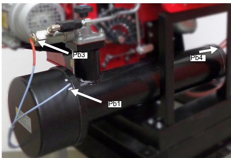
Fig. 8 - Collegamenti sonde Danfoss MCX
