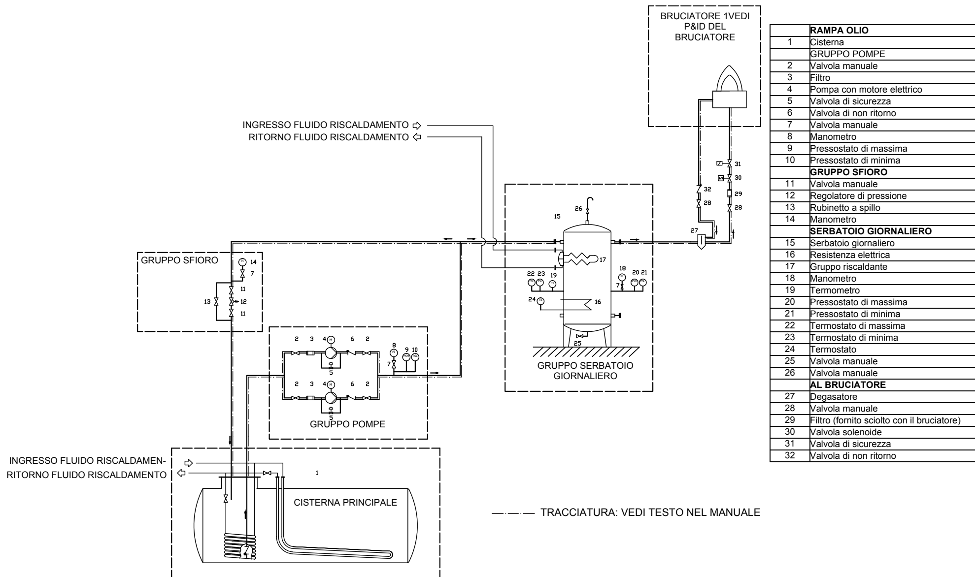
Fig. 6 - 3ID0023 v2 - Schema idraulico - Configurazione per un solo bruciatore
