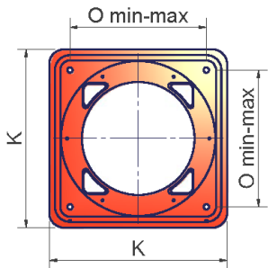
Flangia bruciatore
