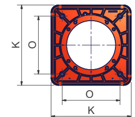
Фланец горелки
