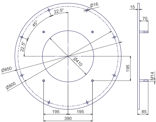
Рекомендуемый контрофланец
