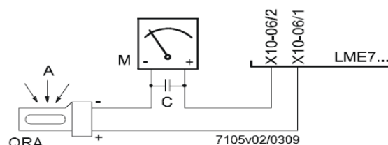
Fig. 19: Rilevazione con fotocellula QRA..
