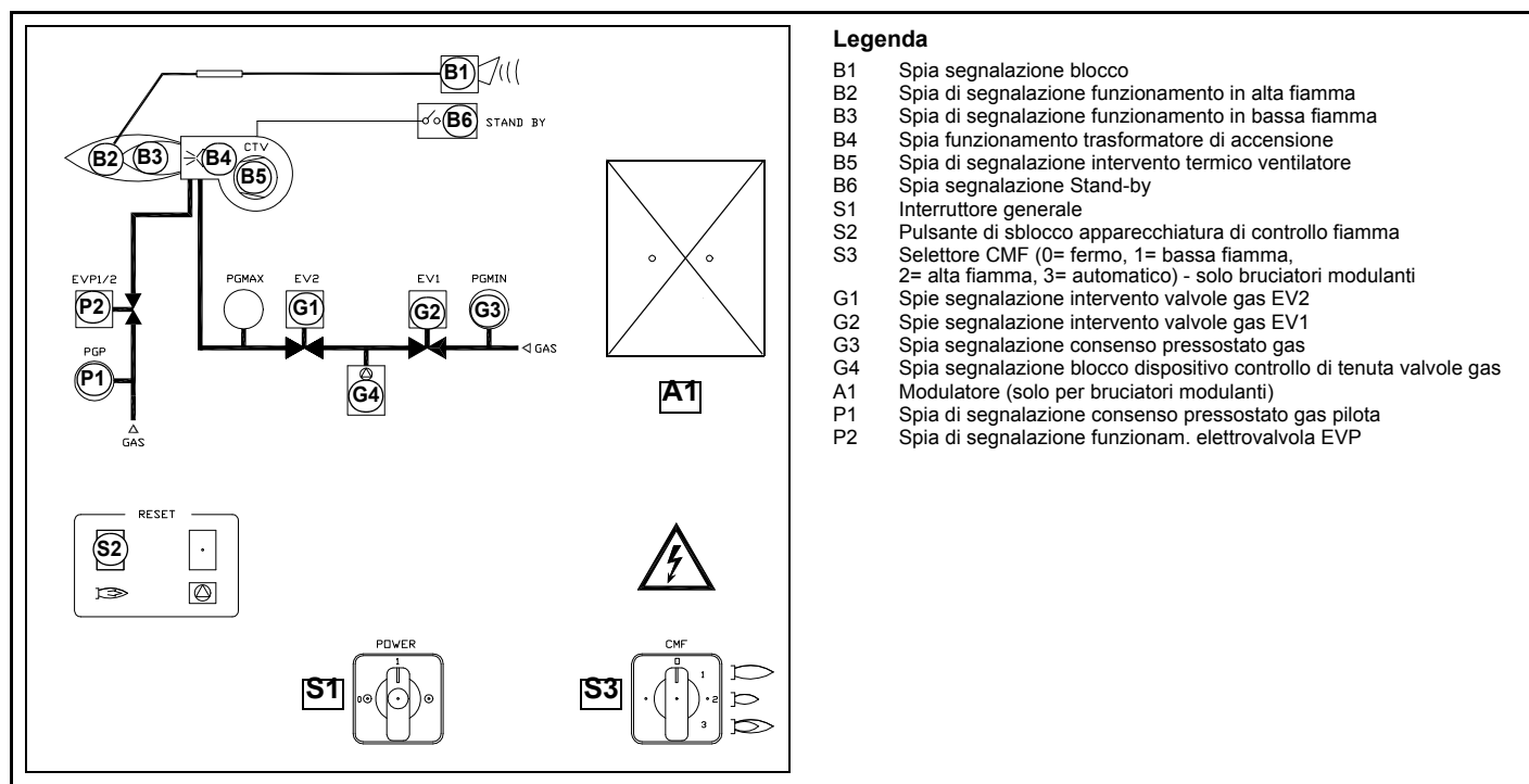
Fig. 10 - Pannello quadro elettrico
