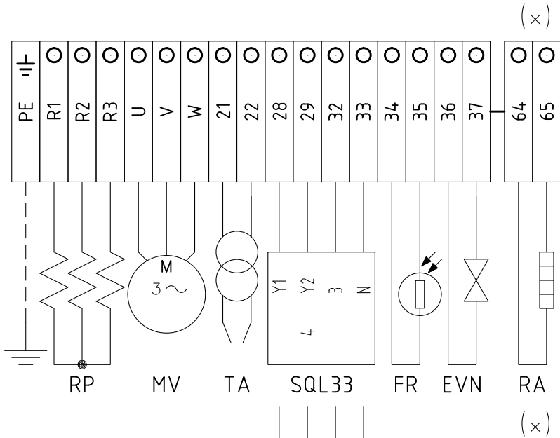
QGG - MC MORSETTIERA COMPONENTI BRUCIATORE BURNER COMPONENT TERMINAL BOARD
