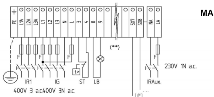
Fig. 2 - Brûleurs modulants
