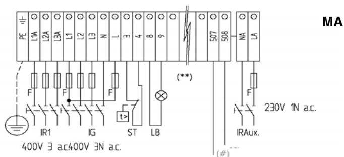
Fig. 2 - Brûleurs modulants
