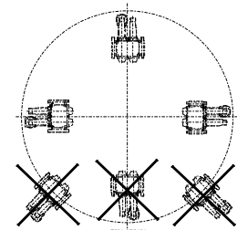
POSIZIONI DI MONTAGGIO SIEMENS VGD..
