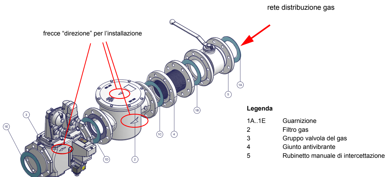
Fig. 4 - Esempio di rampa gas
