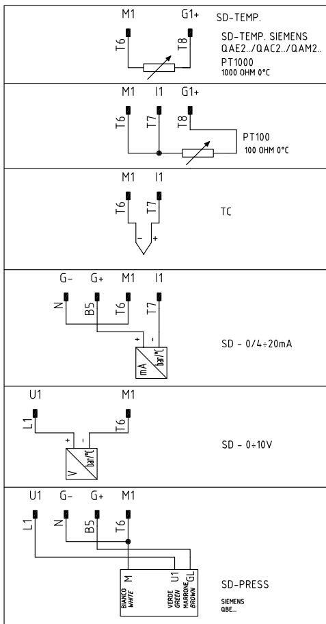
Fig. 17 - Collegamento sonde
