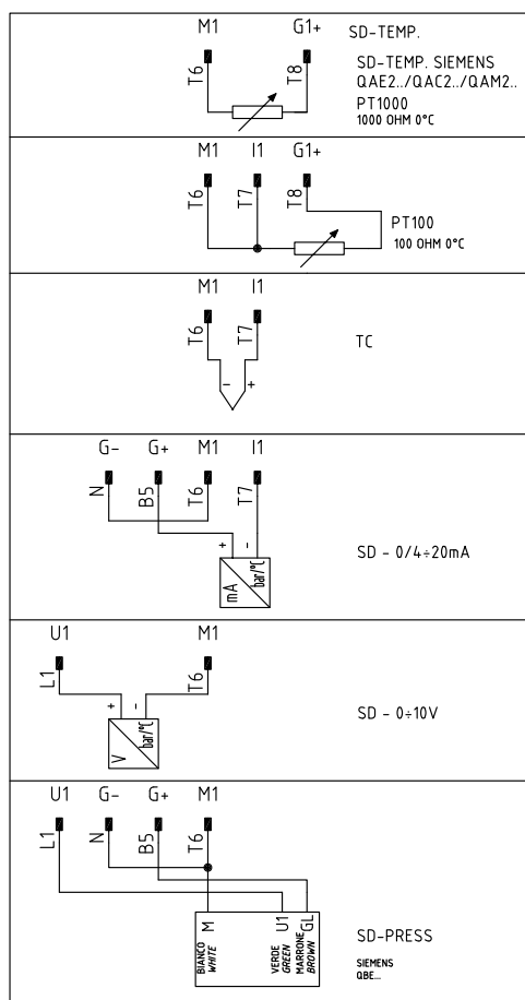
Рис. 18 - - Соединение датчиков
