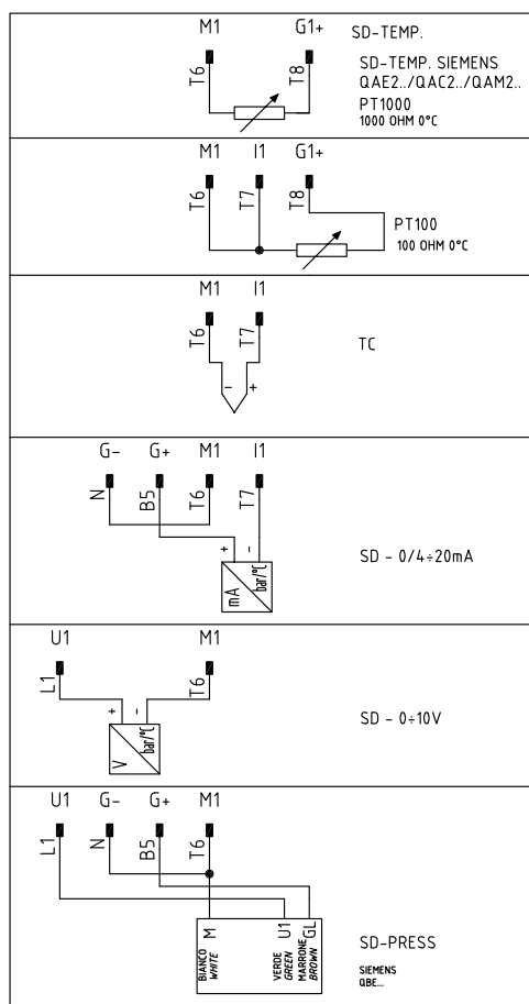
Рис. 18 - - Соединение датчиков
