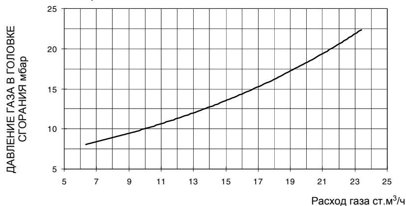
LG550 Горелки на сжиженном газе
