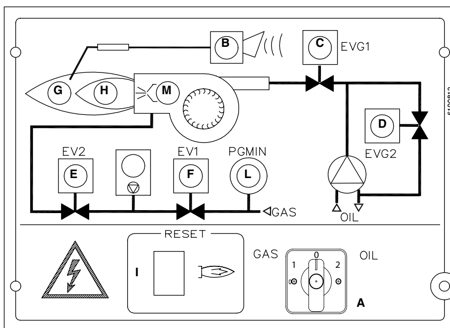
Fig. 18 - Pannello quadro elettrico
