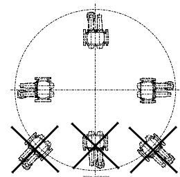
ПОЗИЦИИ ПРИ МОНТАЖЕ SIEMENS VGD..
