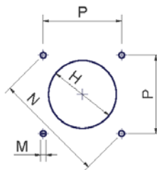
Схема сверления плиты котла
