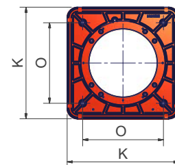
Фланец горелки
