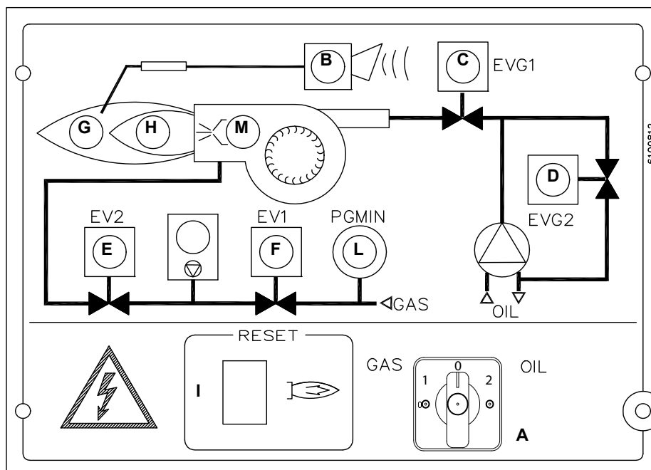
Fig. 15 - Pannello quadro elettrico
