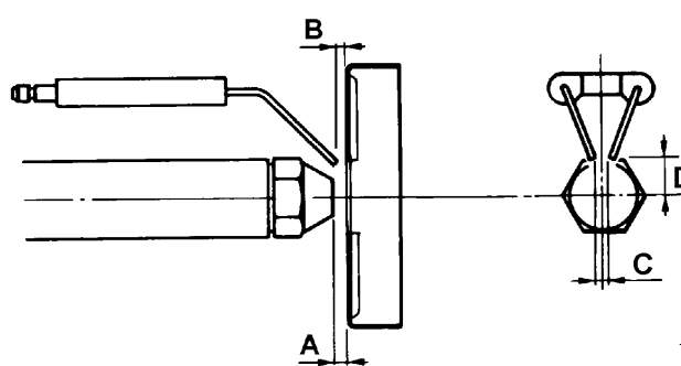
Fig. 21b - Brûleurs G10 et G18
