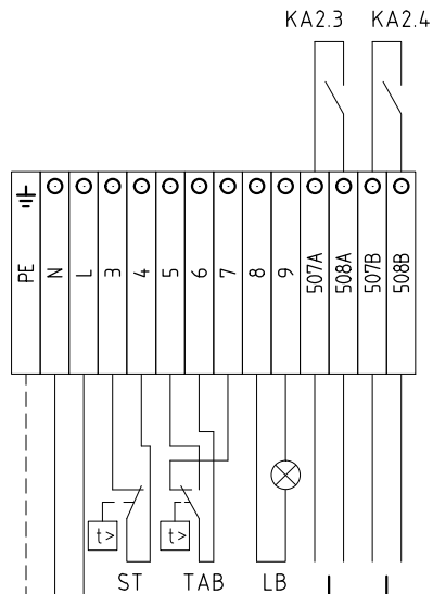
QUADRO QG – MORSETTIERA MA2 MORSETTIERA ALIMENTAZIONE - PIASTRA 2 SUPPLY TERMINALS - PLATE 2
