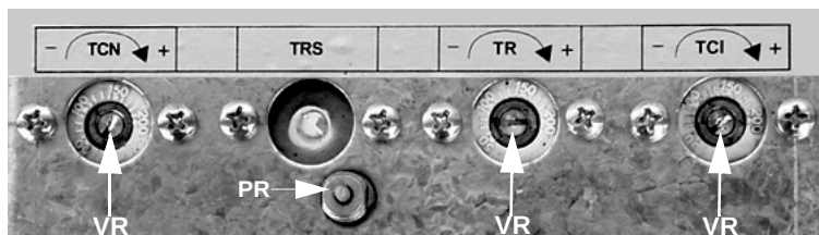
Fig. 9b - Bruciatori a nafta densa
