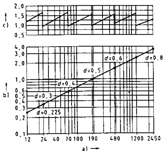
Fig. 8 - Carico termico, diametro e lunghezza del focolare di prova in funzione della potenza bruciata Q.
