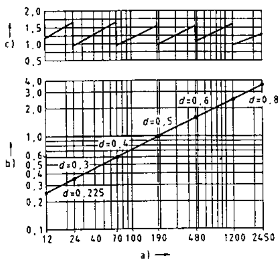
Fig. 8 - Carico termico, diametro e lunghezza del focolare di prova in funzione della potenza bruciata Q.
