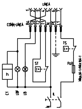
Fig. 19: Quemadores de 1 etapa
