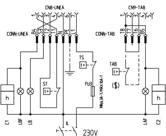
Fig. 20: Quemadores 2 etapas
