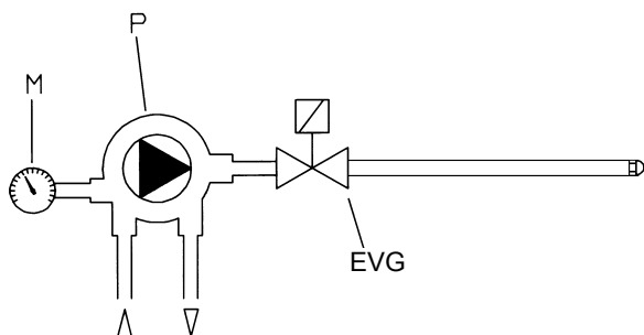
Fig. 30 - Quemadores 1 etapa
