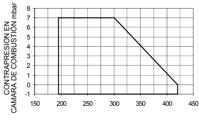
LO400 Monoetapicos
