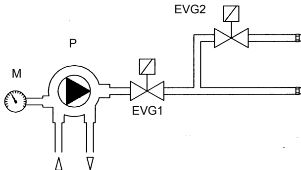
Fig. 31 - Quemadores 2 etapas
