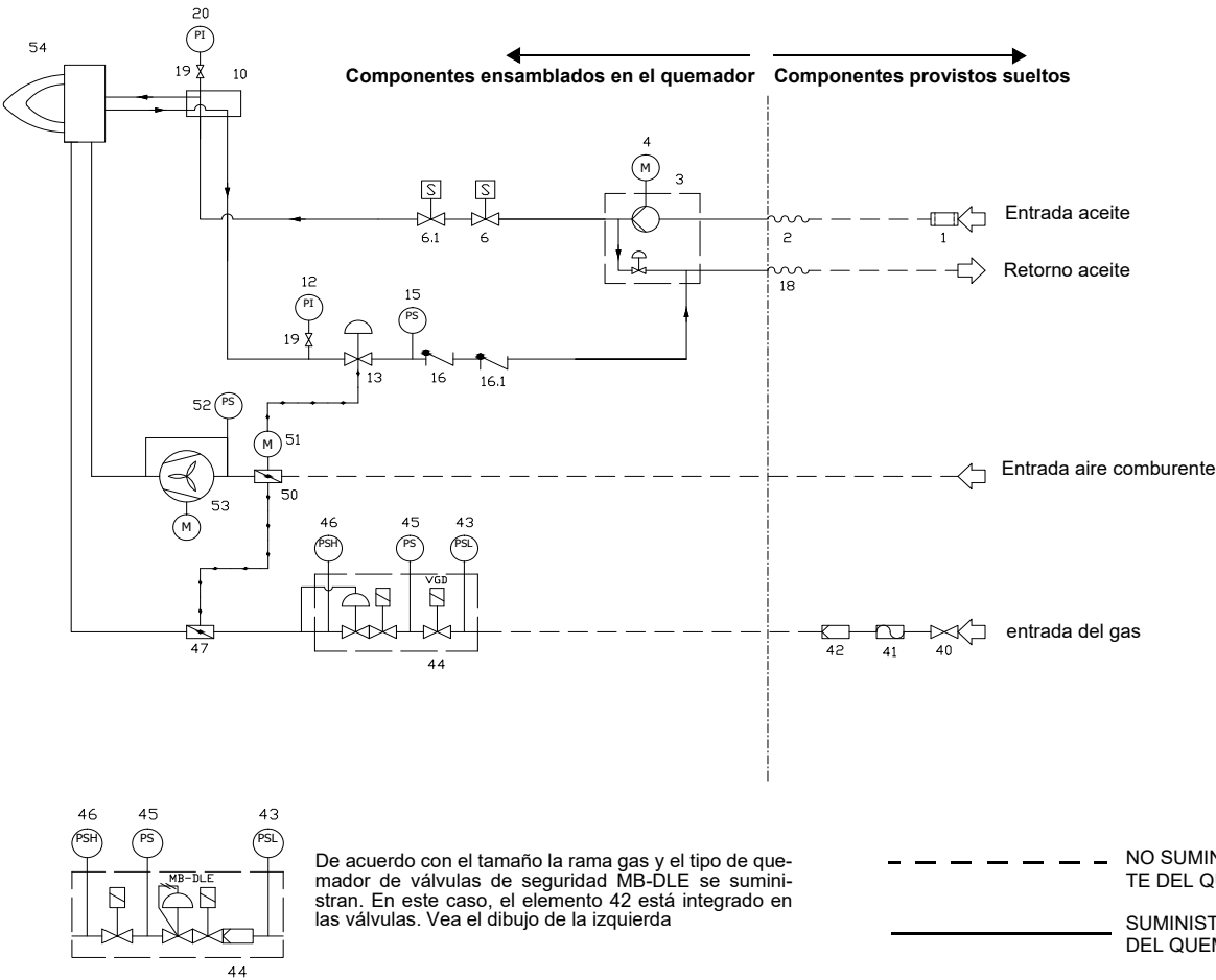
Fig. 2 - 3I2MG-09 v1 Esquema hidráulico
