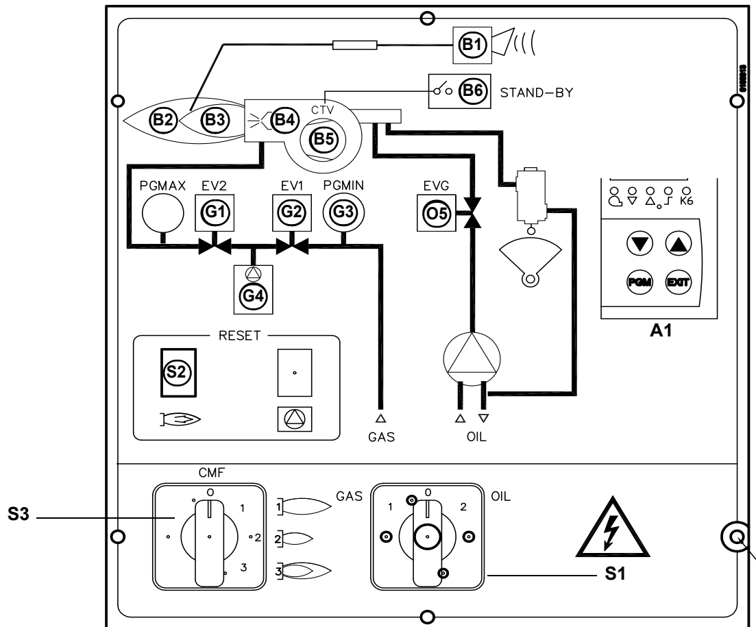
Fig. 3 - Pannelo cuadro electrico
