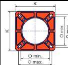
Brida quemador
