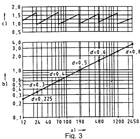
Fig.3:Potencia térmica, diámetro y longitud del hogar de prueba en función de la potencia quemada in kW.
