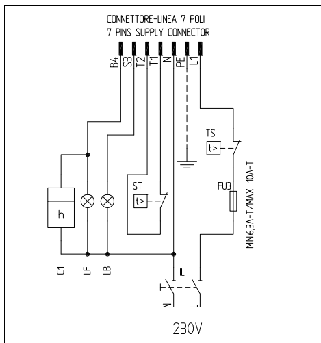
Fig. 23 - Conector 7-polos
