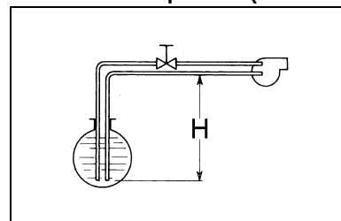
Instalación en aspiración (dos tubos)
