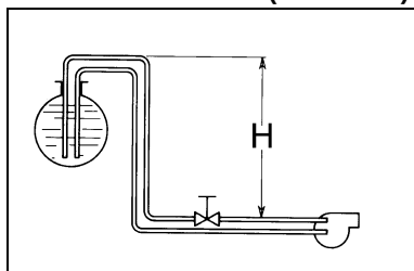
Instalación de sifón (dos tubos)
