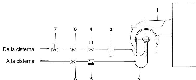
Fig. 10 - Sistema bitubo
