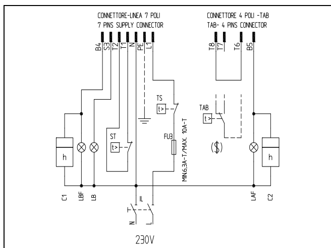
Fig. 9 Conectores 7 y 4 polos
