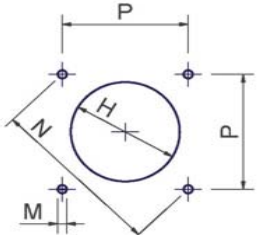
Plantilla de perforación recomendada de la placa de la caldera.
