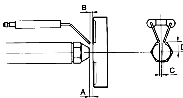
Fig. 21b - Bruciatori G10 e G18
