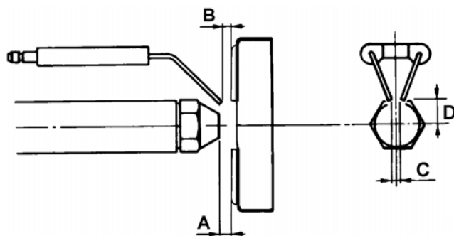
Fig. 21a - Bruciatori G4 e G6
