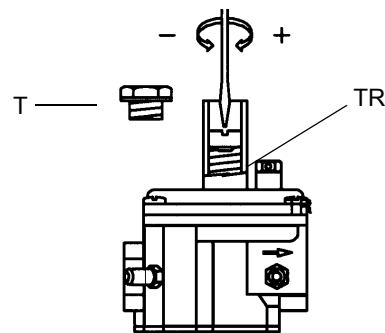
Stabilizzatore di pressione
