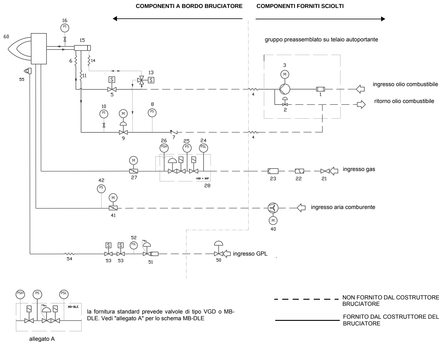
Fig. 3 - 3I2MG71 v0 Schema idraulico - ugello tipo M3
