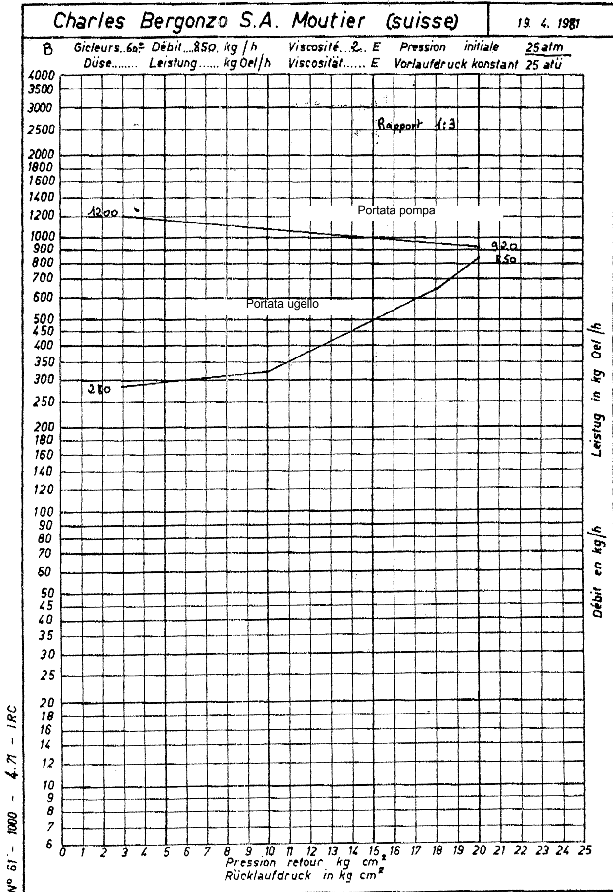
Fig. 18 - Ugello Bergonzo B- Esempio con ugello da 850 kg/h
