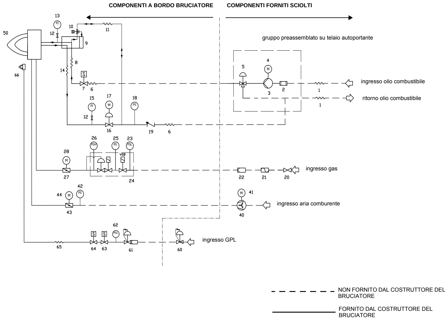
Fig. 4 - 3I2MG72 v0 Schema idraulico - ugello tipo G
