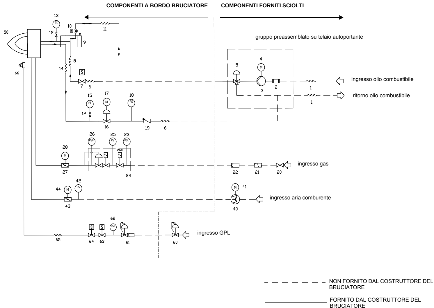
Fig. 4 - 3I2MG72 v0 Schema idraulico - ugello tipo G
