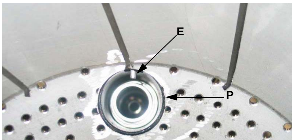
Fig. 25 - Particolare del diffusore con pilota (P) e elettrodo di accensione (E)
