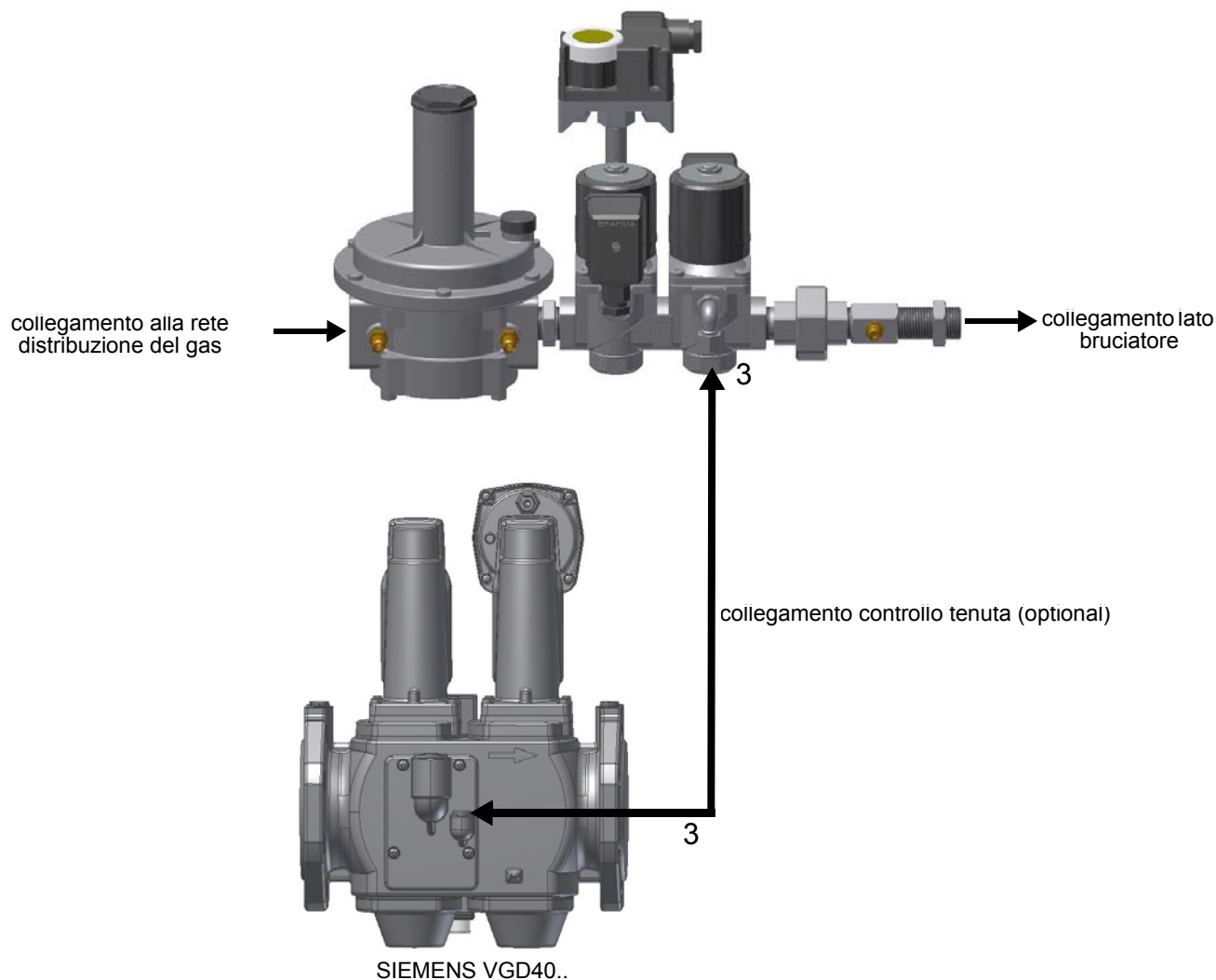
Fig. 6 - attacco (3) tubetto da rampa pilota al gruppo valvole della rampa principale (nello schema non è previsto ma si può eseguire)
