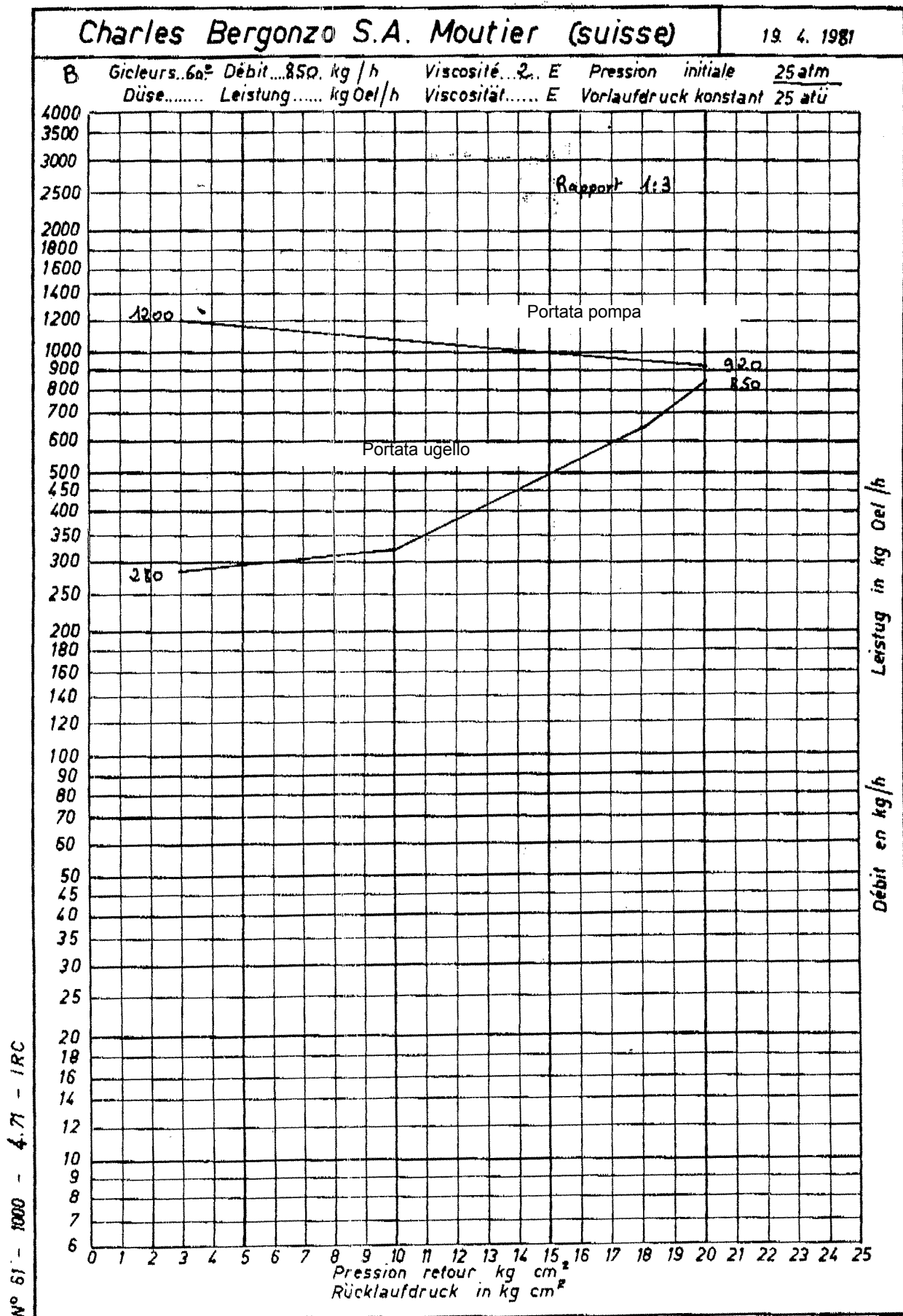
Fig. 18 - Ugello Bergonzo B- Esempio con ugello da 850 kg/h
