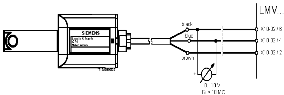
Fig. 28 - Rilevazione con fotocellula QRI..
