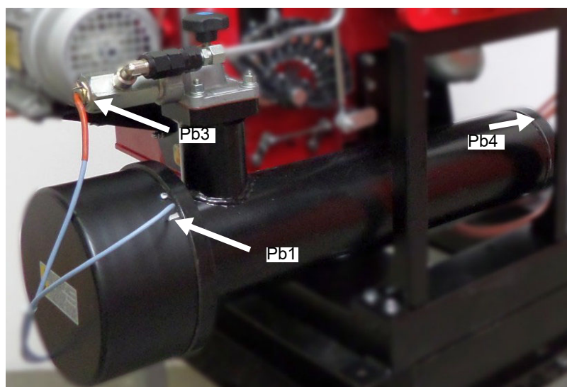
Fig. 12 - Collegamenti sonde Danfoss MCX
