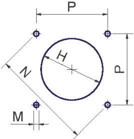
Foratura caldaia
