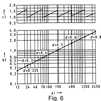
Fig. 6 - Carico termico, diametro e lunghezza del focolare di prova in funzione della potenza bruciata in kW
