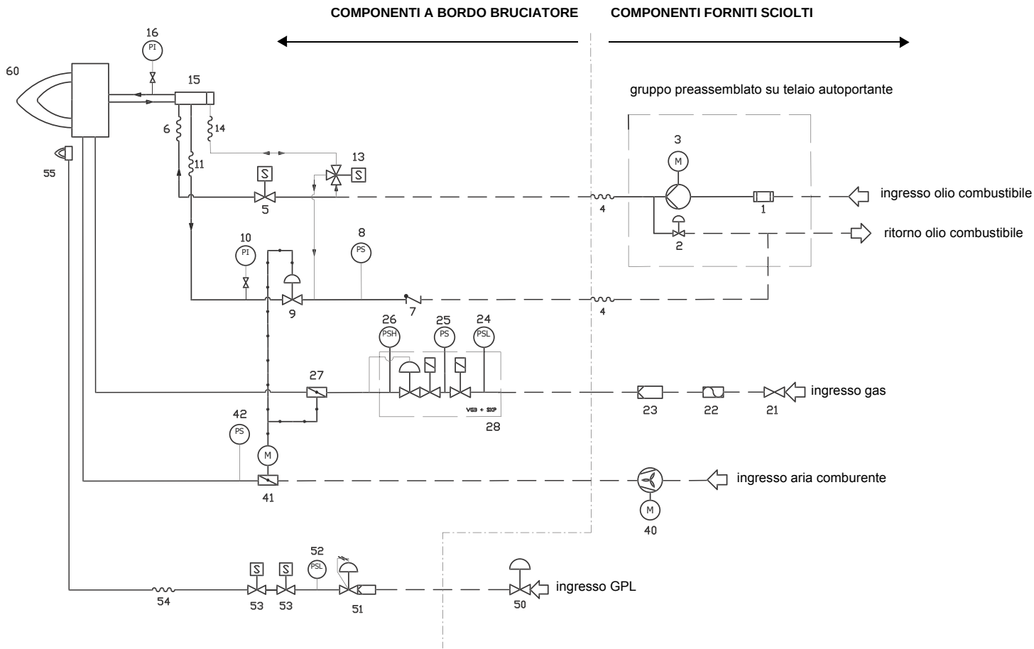
Fig. 3 - 3I2MG51 v1 Schema idraulico - ugello tipo M3
