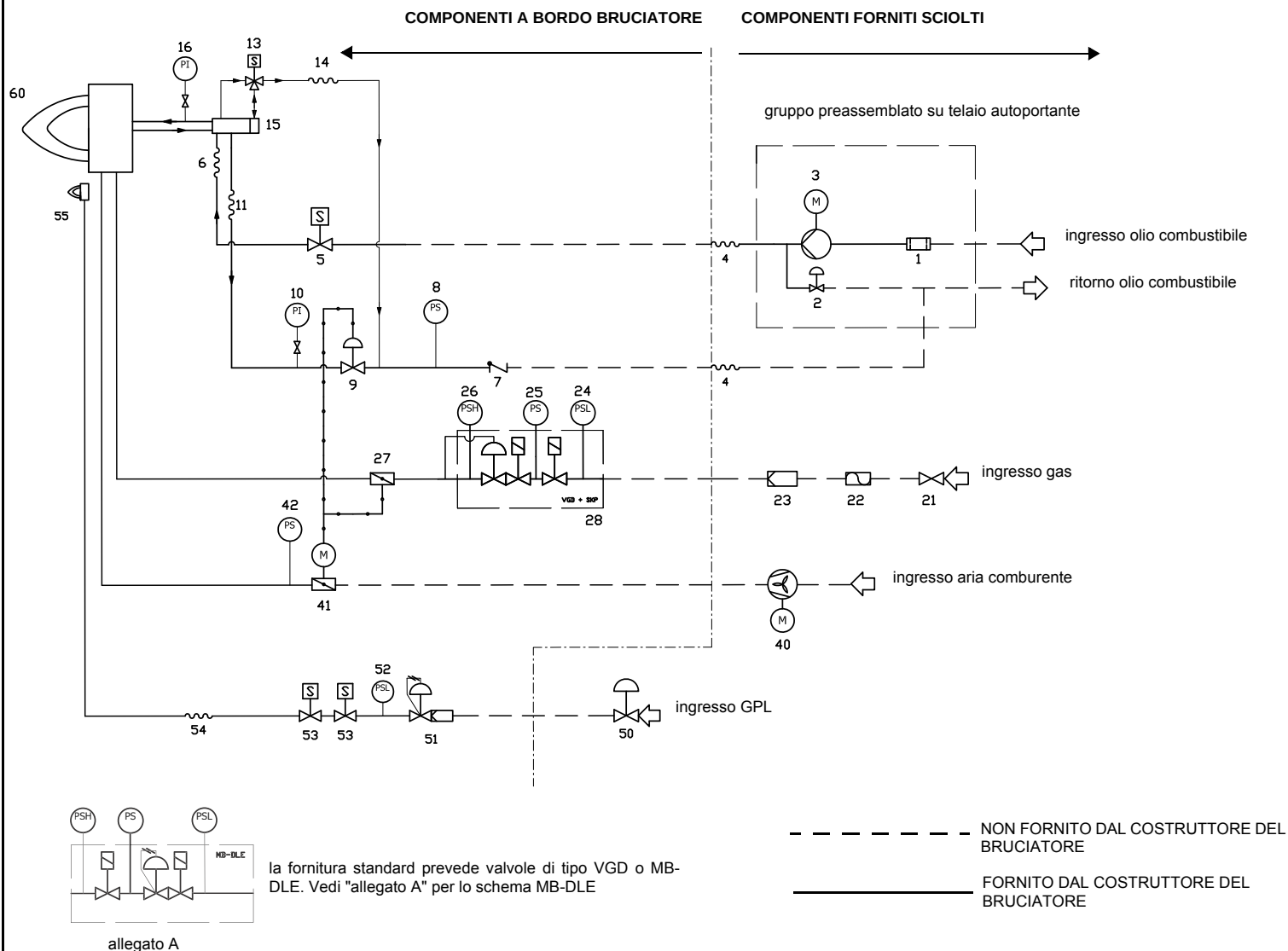
Fig. 4 - 3I2MG52 v0 Schema idraulico - ugello tipo G
