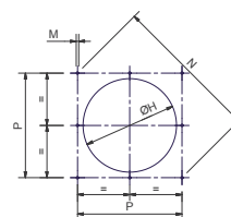
Perçage de la chaudière recommandé
