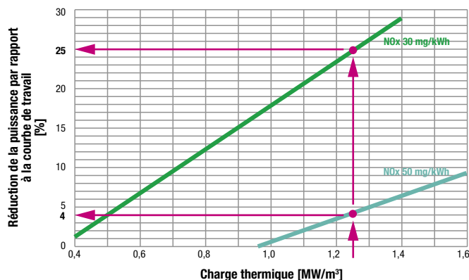
RÉDUCTION DE LA PUISSANCE PAR RAPPORT À LA COURBE DE FONCTIONNEMENT DU BRÛLEUR
