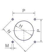
Perçage de la chaudière recommandé
