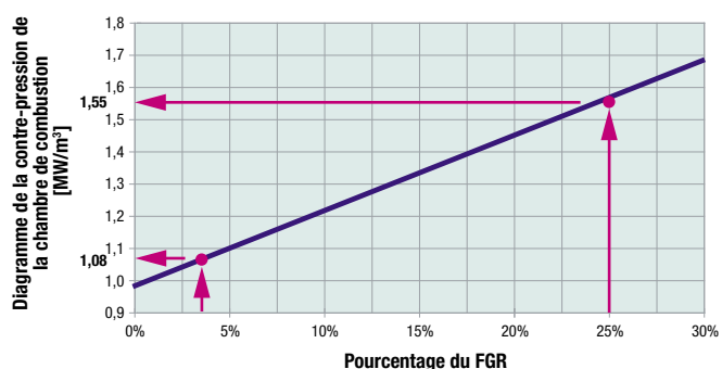
DIAGRAMME D'AUGMENTATION DE LA CONTRE-PRESSION DE LA CHAMBRE DE COMBUSTION
