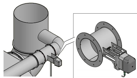
Clapet supplémentaire sur la cheminée version avec servomoteur (option 1)
