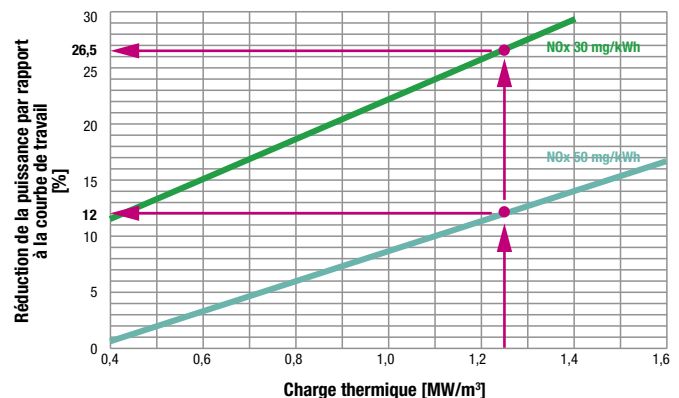
RÉDUCTION DE LA PUISSANCE PAR RAPPORT À LA COURBE DE FONCTIONNEMENT DU BRÛLEUR
