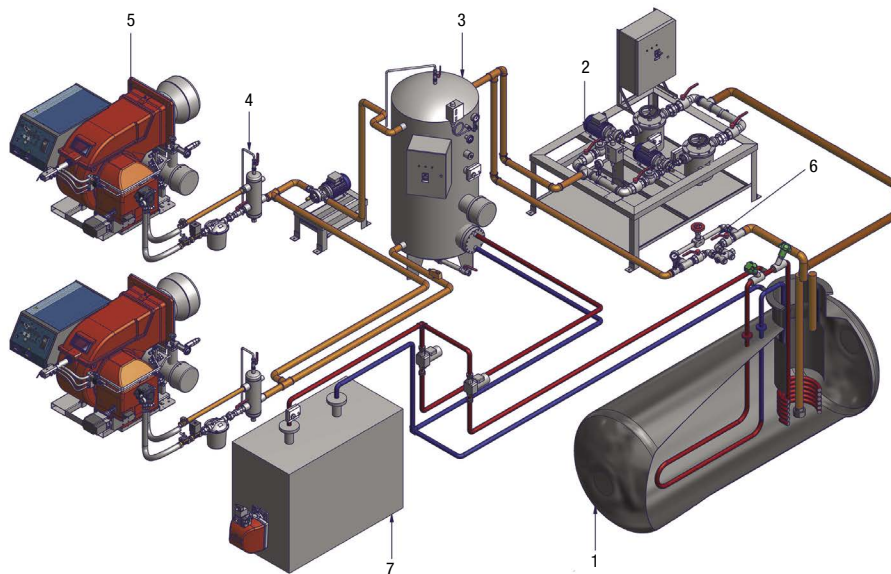
Sch. 02 - Exemple de circuit pour brûleurs à fioul avec pulvérisation pneumatique.
