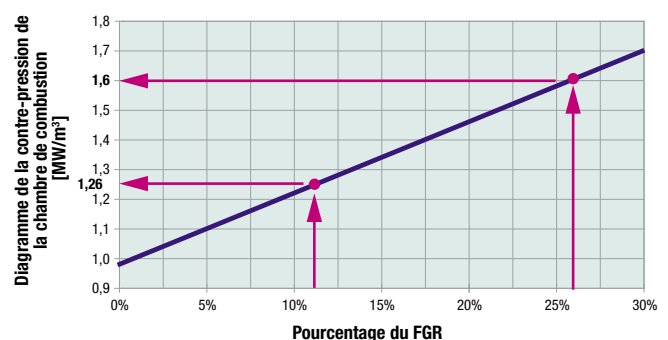
DIAGRAMME D'AUGMENTATION DE LA CONTRE-PRESSION DE LA CHAMBRE DE COMBUSTION
