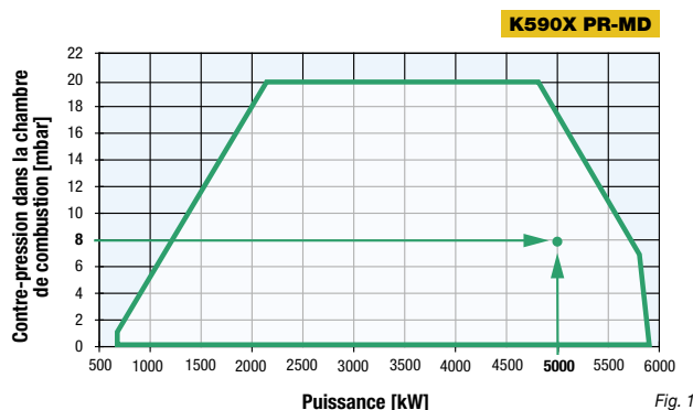
COURBE DE FONCTIONNEMENT DU BRÛLEUR
