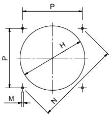
Perçage de la chaudière recommandé
