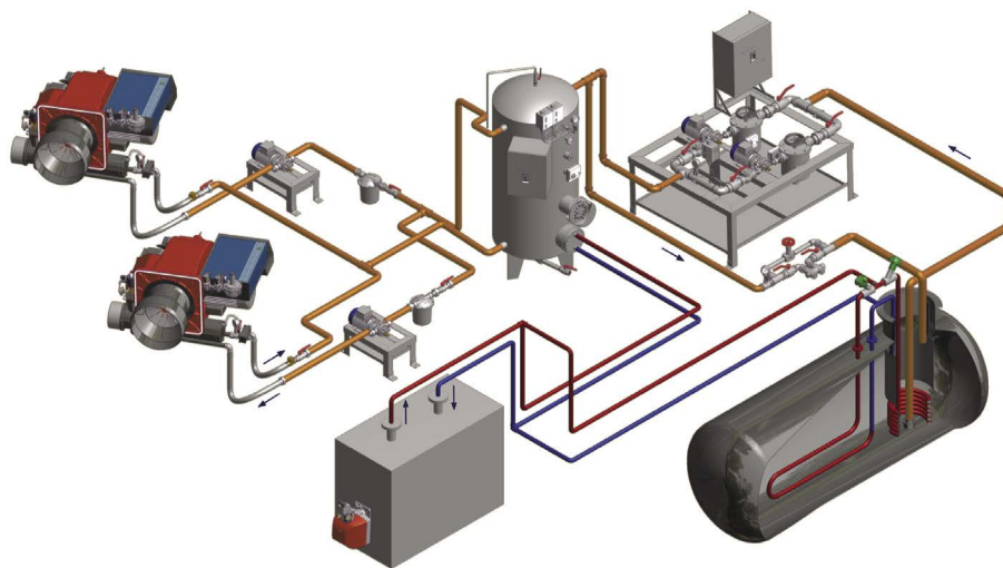
Sch. 02 - Exemple de circuit pour brûleurs à fioul avec pulvérisation pneumatique.
