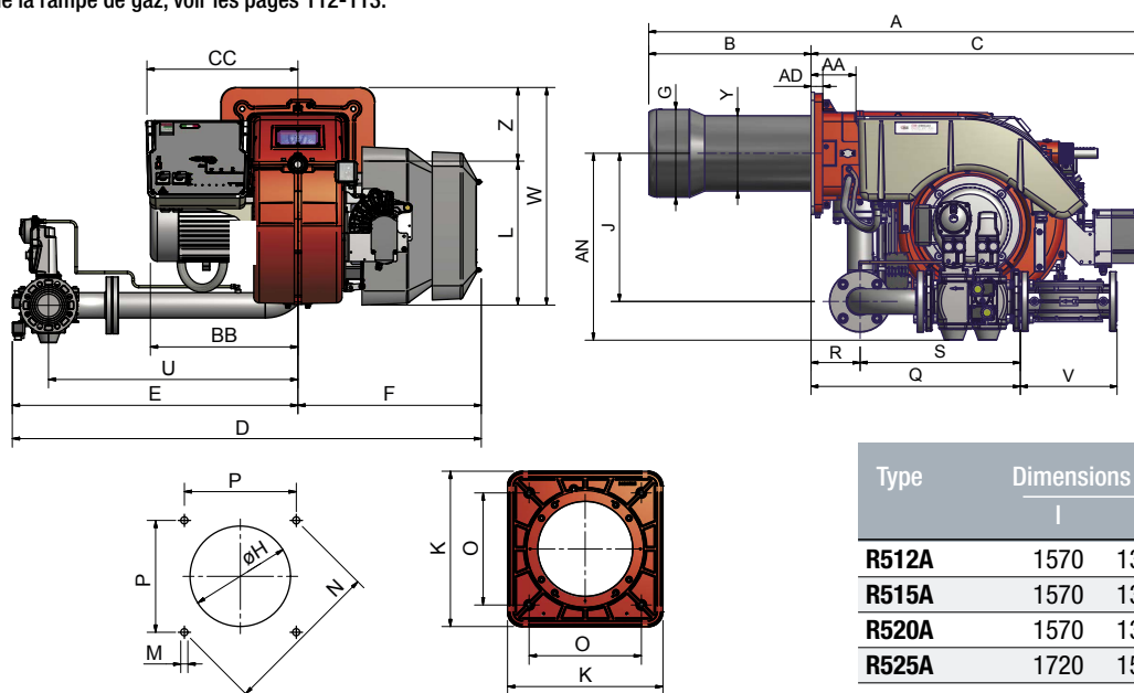
Perçage de la chaudière recommandé
