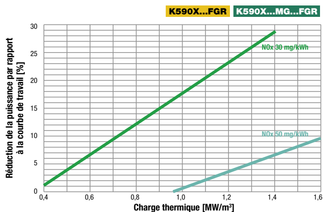
RÉDUCTION DE LA PUISSANCE PAR RAPPORT À LA COURBE DE FONCTIONNEMENT DU BRÛLEUR
