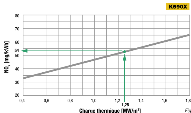
DIAGRAMME NO x EN RELATION AVEC LA CHARGE THERMIQUE DE LA CHAUDIÈRE
