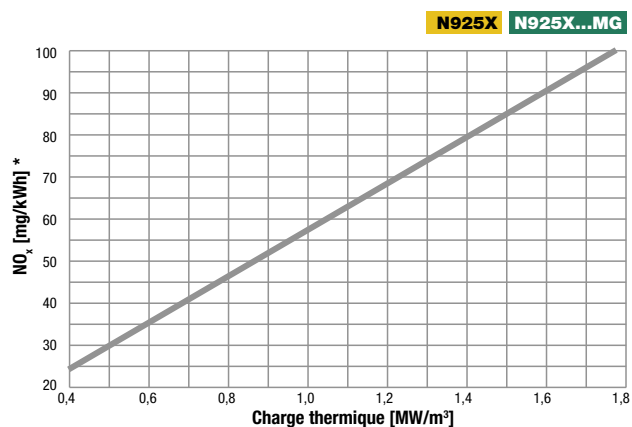
DIAGRAMME NO x EN RELATION AVEC LA CHARGE THERMIQUE DE LA CHAUDIERE
